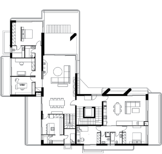
κάτοψη 2ου ορόφου
